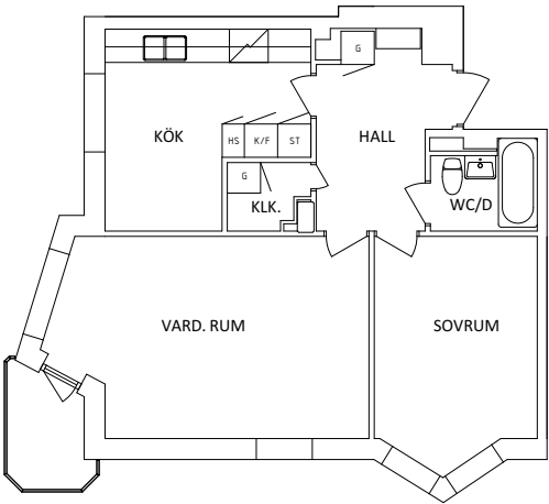
Befintlig planritning
