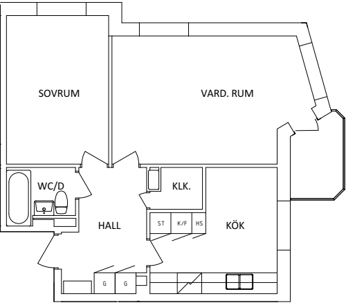
Befintlig planritning
