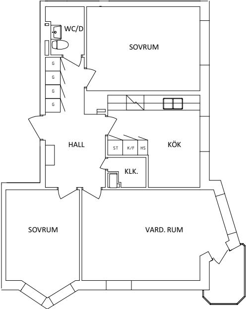
Befintlig planritning
