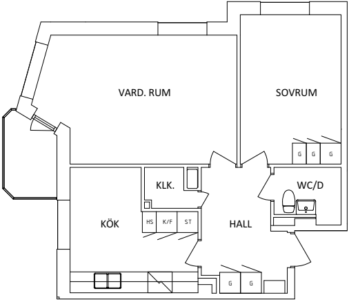
Befintlig planritning
